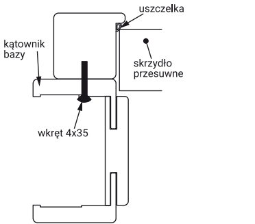
rys. 8 - Zamocowanie belki odbojowej do kątownika bazy
