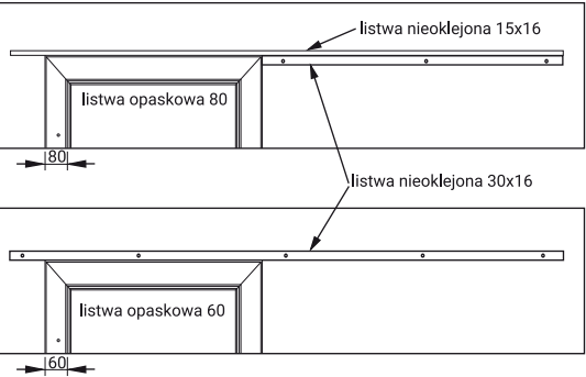
rys. 5 - Porównanie montażu listw nieoklejonych wyrównujących przy opaskach „60” oraz „80”
