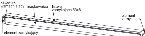
rys. 1 - Złożenie maskownicy z elementami zamykającymi
