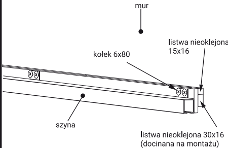
rys. 6 - Montaż szyny do ściany (widok dla opaski 80)
