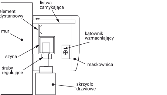
rys. 4 - Regulacja śrub, zakończenie montażu
