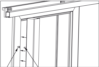
rys. 9 - Montaż belki do zabudowanego tunelu
