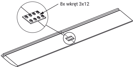
rys. 10 - Połączenie maskownicy w przypadku systemu podwójnego
